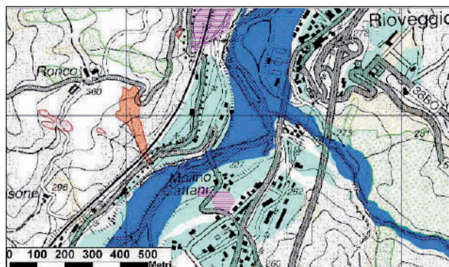
FIGURA 39 - Carta delle frane della zona circostante la frana di Ronco Puzzola, circa 700 m a ESE dell'abitato di Rioveggio
