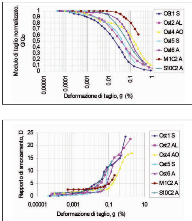
FIGURA 7 - Curve di decadimento espresse come rapporto G/G_0 e curve dello smorzamento D (%), entrambe in funzione dello sforzo di taglio applicato
