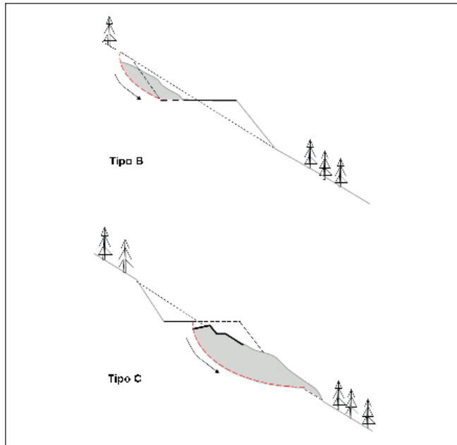
FIGURA 6 – Tipiche situazioni di innesco di movimenti di frane che interessano la viabilità appenninica
