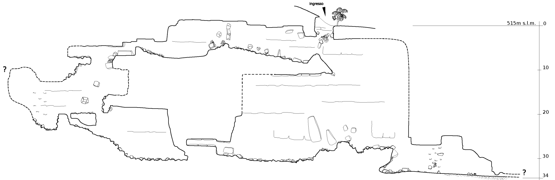
SEZIONE LONGITUDINALE
